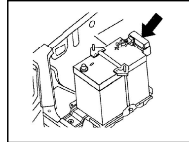
جعبه فیوز شماره 3 : جعبه فیوز داخل محفظه موتور، سمت راست باتری قرار دارد.
